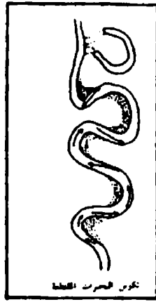
تكوين البحيرات المنقطعة
